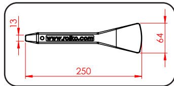
Plastdækjern til en skånsom montering af Pu-/luftdæk på fælg | Plastic tyre lever for a gentle assembly of PU and pneumatic tyres on rims
